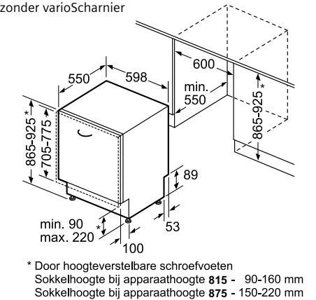
SX-modellen zonder varioScharnier
