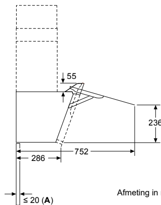
Afmeting in mm Apparaat in luchttafvoermodus
