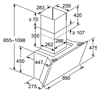
Afmeting in mm Apparaat in luchtafvoermodus
