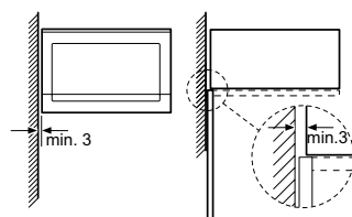
Afmetingen in mm
