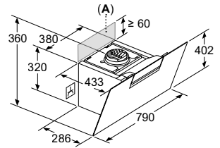
Afmeting in mm Apparaat in luchtcirculatiemodus zonder kanaal
