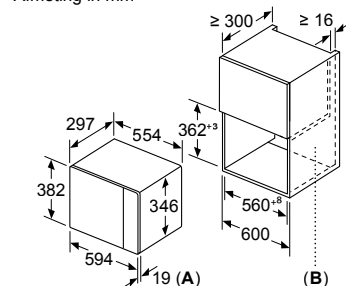
A: 20 mm voor metalen front B: Achterwand open
