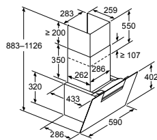
Afmeting in mm Apparaat in luchttafvoermodus
