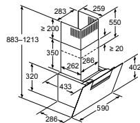
Afmeting in mm Apparaat in luchtcirculatiemodus
