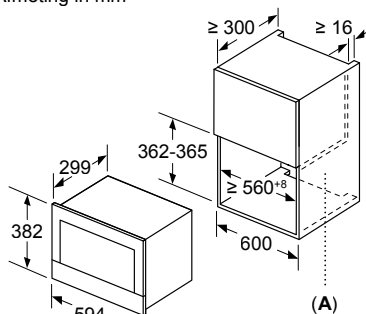
A: Achterwand open
