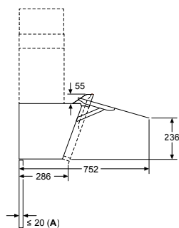
Afmeting in mm Apparaat in luchttafvoermodus
