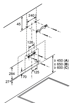
Afmeting in mm Wandinstallatie met luchtkanaal
