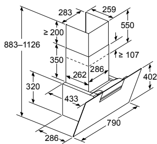
Afmeting in mm Apparaat in luchttafvoermodus
