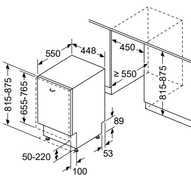
SR-modellen met varioScharnier
