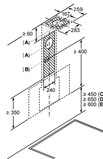
Afmeting in mm Apparaat in luchtcirculatiemodus zonder kanaal
