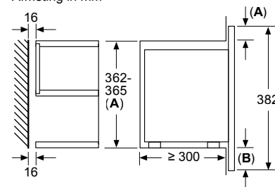
A: Overstek boven: Nis 362: 6 mm Nis 365: 3 mm B: Overstek onder: 14 mm
